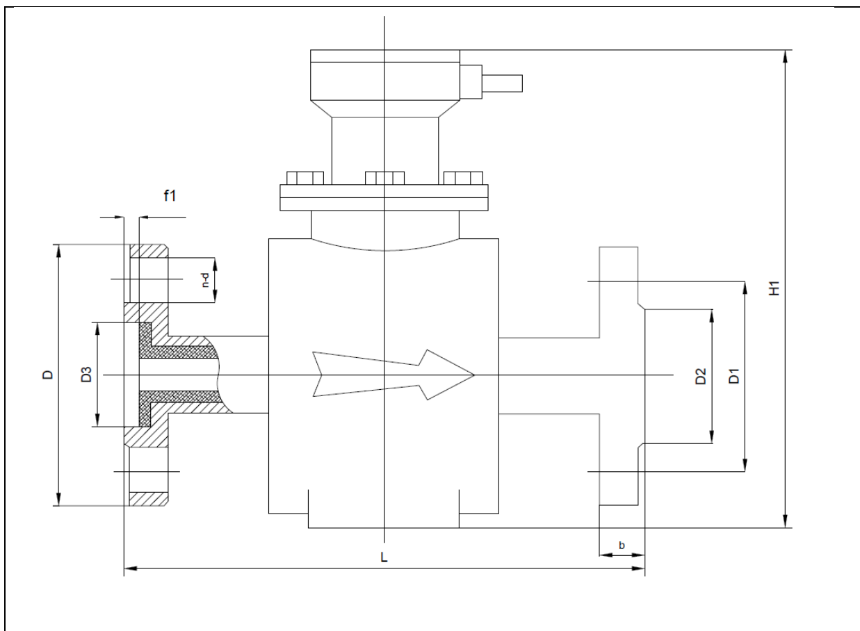
Рис.6. Схема раздельного электромагнитного расходомера
