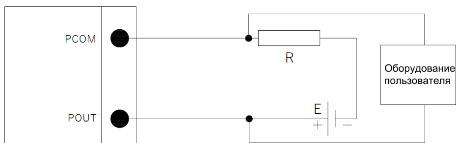
Частотный (импульсный) выход
