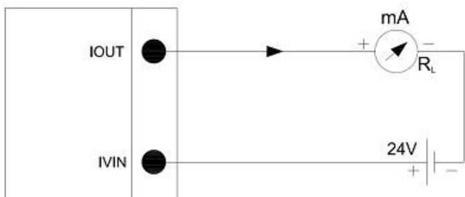
Токовый выход (пассивный) - двухпроводное соединение
