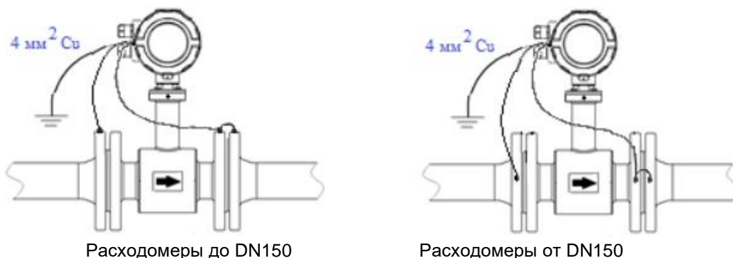
Рис.5. Схемы заземления для расходомеров.
