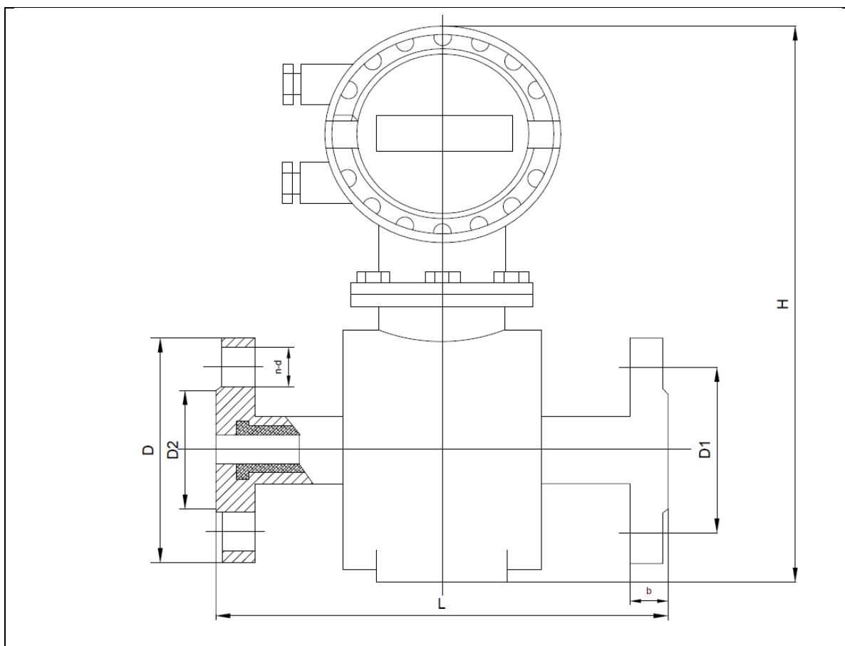
Рис.5. Схема компактного электромагнитного расходомера
