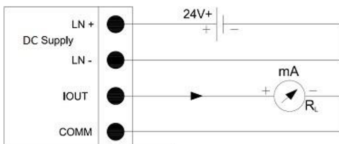
Токовый выход (активный) - четырехпроводное соединение (гальванически развязан)
