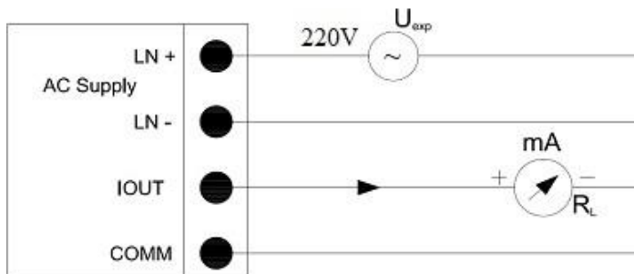
Токовый выход (активный) - четырехпроводное соединение (гальванически развязан)
