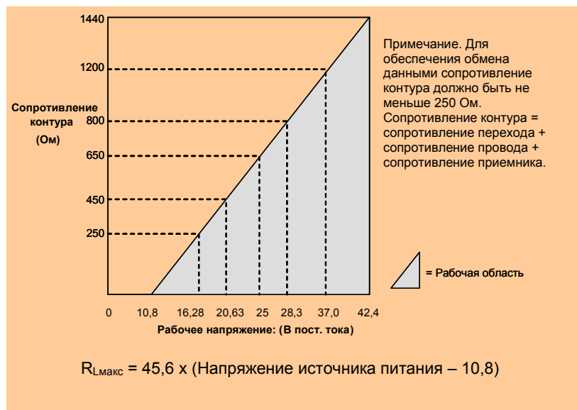
Рисунок 3. График и расчеты зависимости сопротивления контура от напряжения питания
