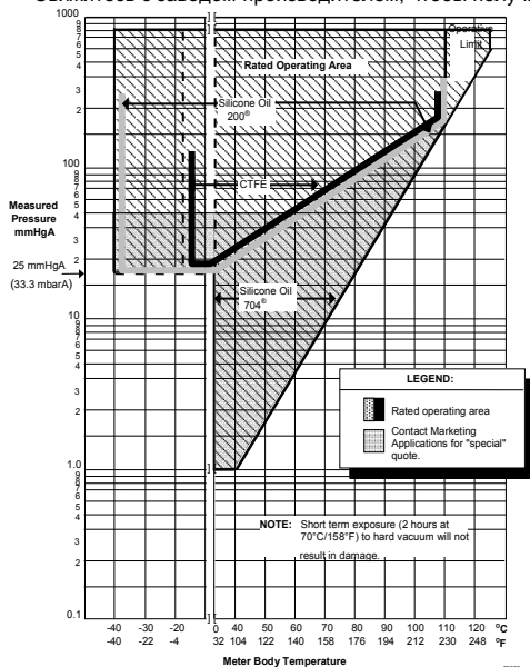
Рисунок 2. График зависимости давления от температуры сенсора
